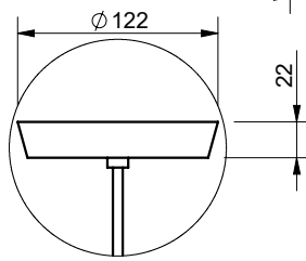
DETALHE A
