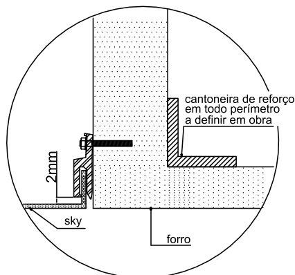
DETALHE 1 s/esc.
