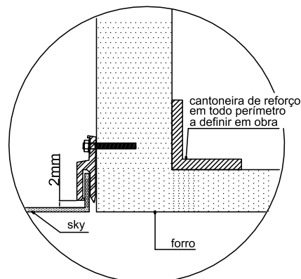
DETALHE 1 s/esc.
